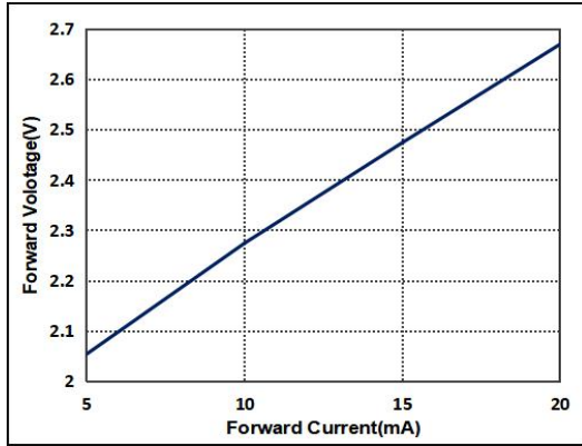
图 3. 典型的电流与电压的关系图
