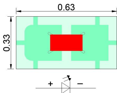
正视图
