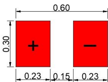
推荐灯珠焊盘设计图
