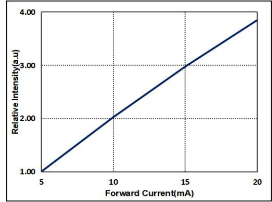
图 4. 典型的输出光通量与电流关系图
