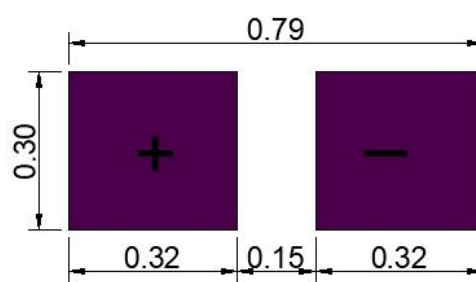
推荐 PCB 焊盘设计图
