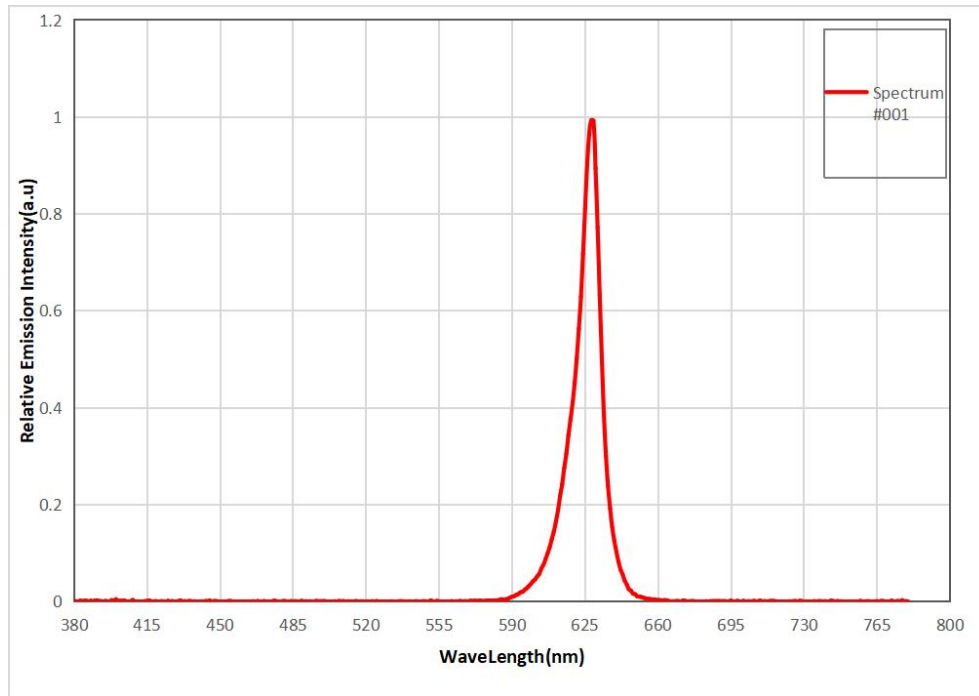
图1. 典型的光功率与光谱分布图
