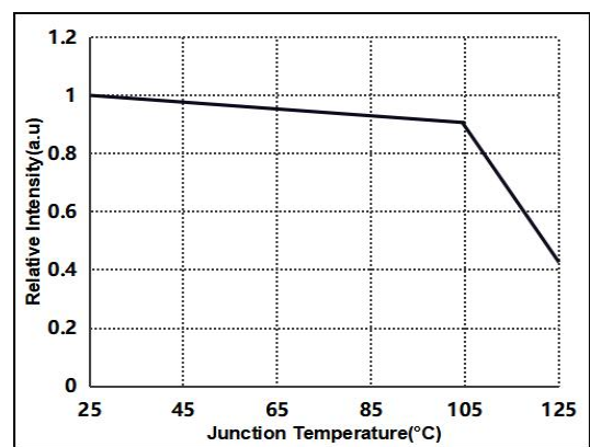
图 6. 输出光通量与结温的关系图
