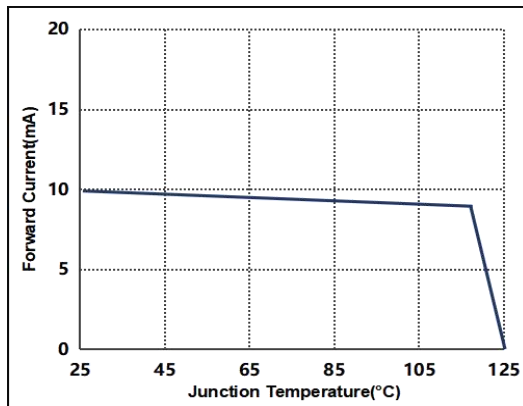
图 5. 电流与结温的关系图
