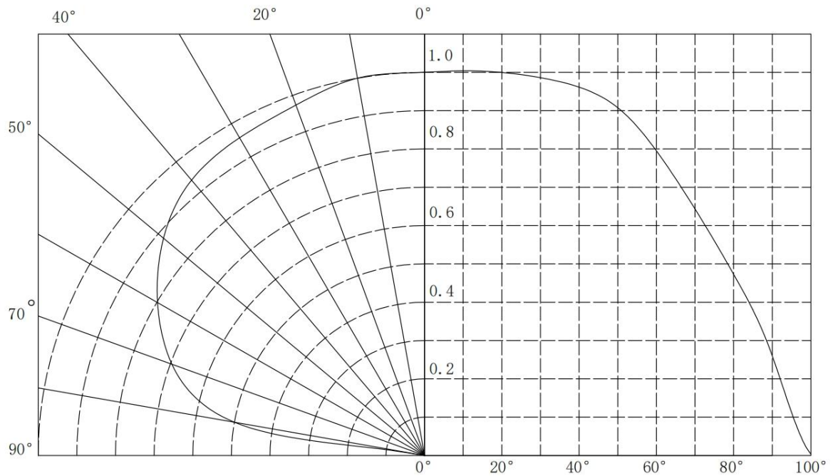
图2. 典型的角分布图
