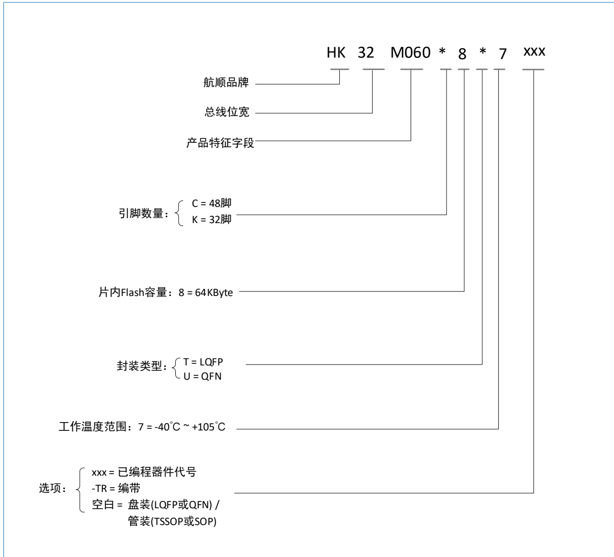
图 8-1 订货代码
