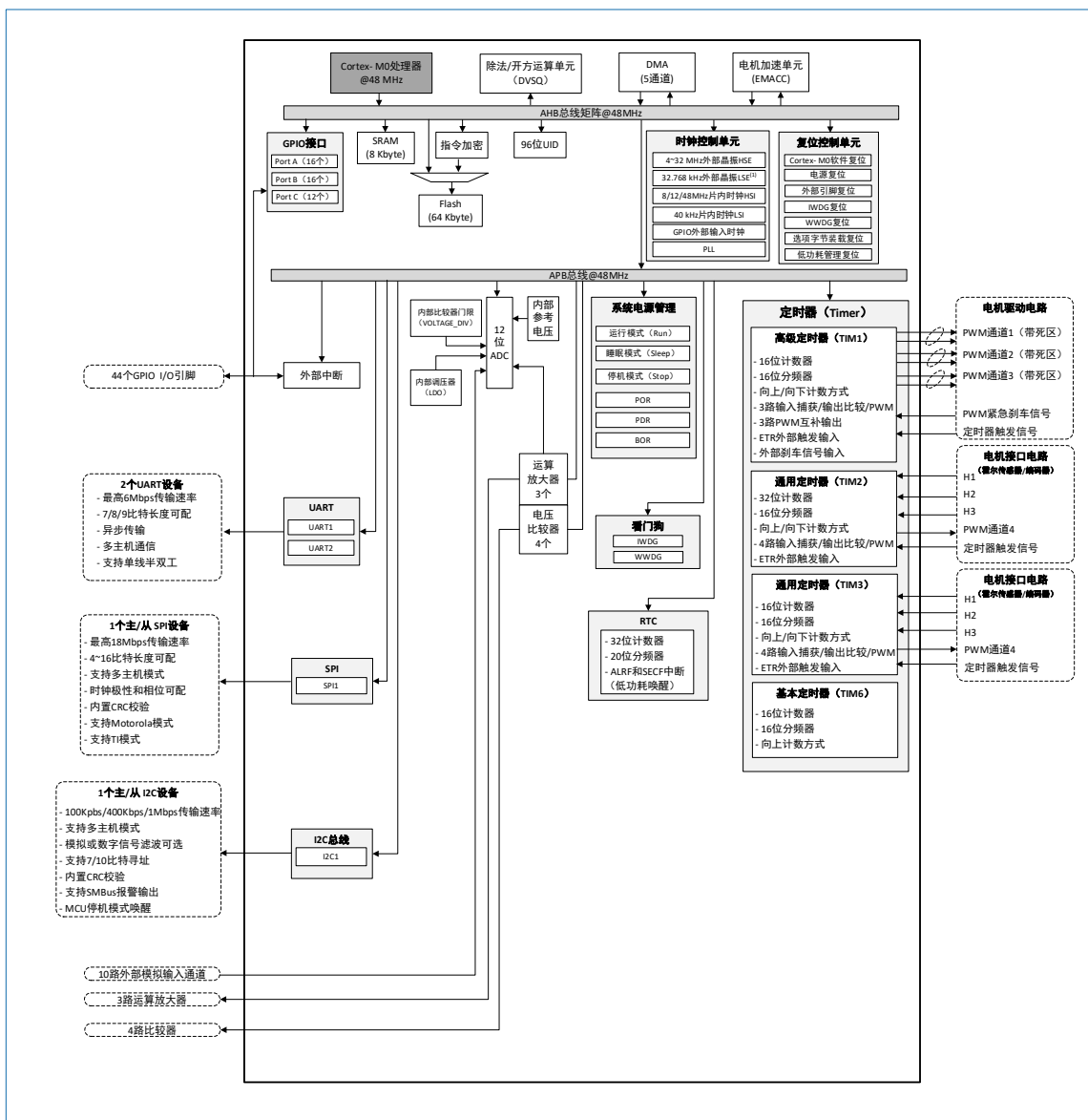
图 3-1 HK32M060C8T7 功能框图
