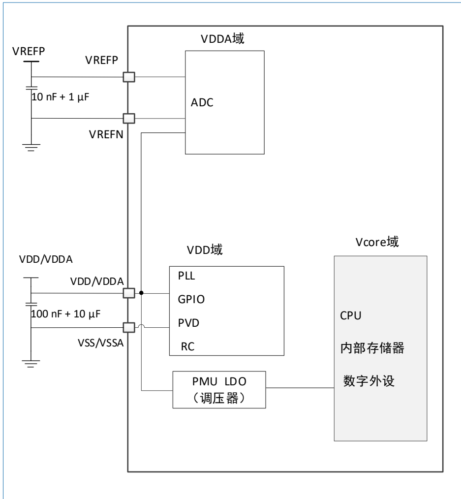
图 5-1 电源框图
