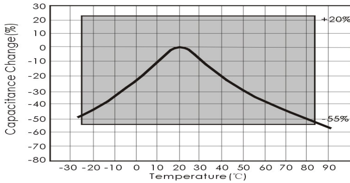
Char:E (Y5U)
